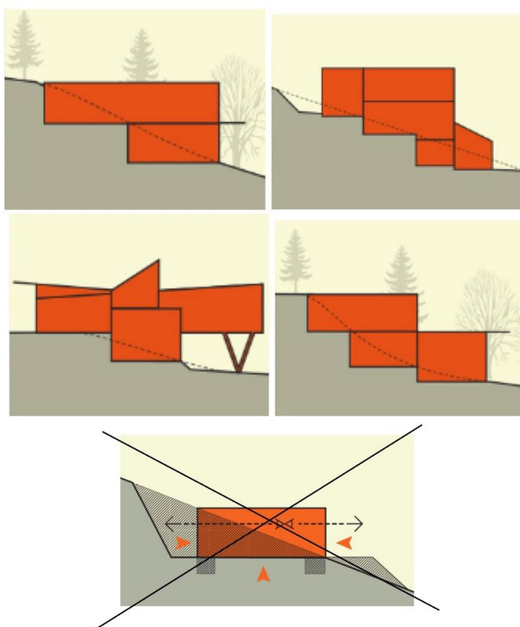
Exemples d'implantation qui limitent les mouvements de sols, le dernier exemple n'est pas autorisé.
